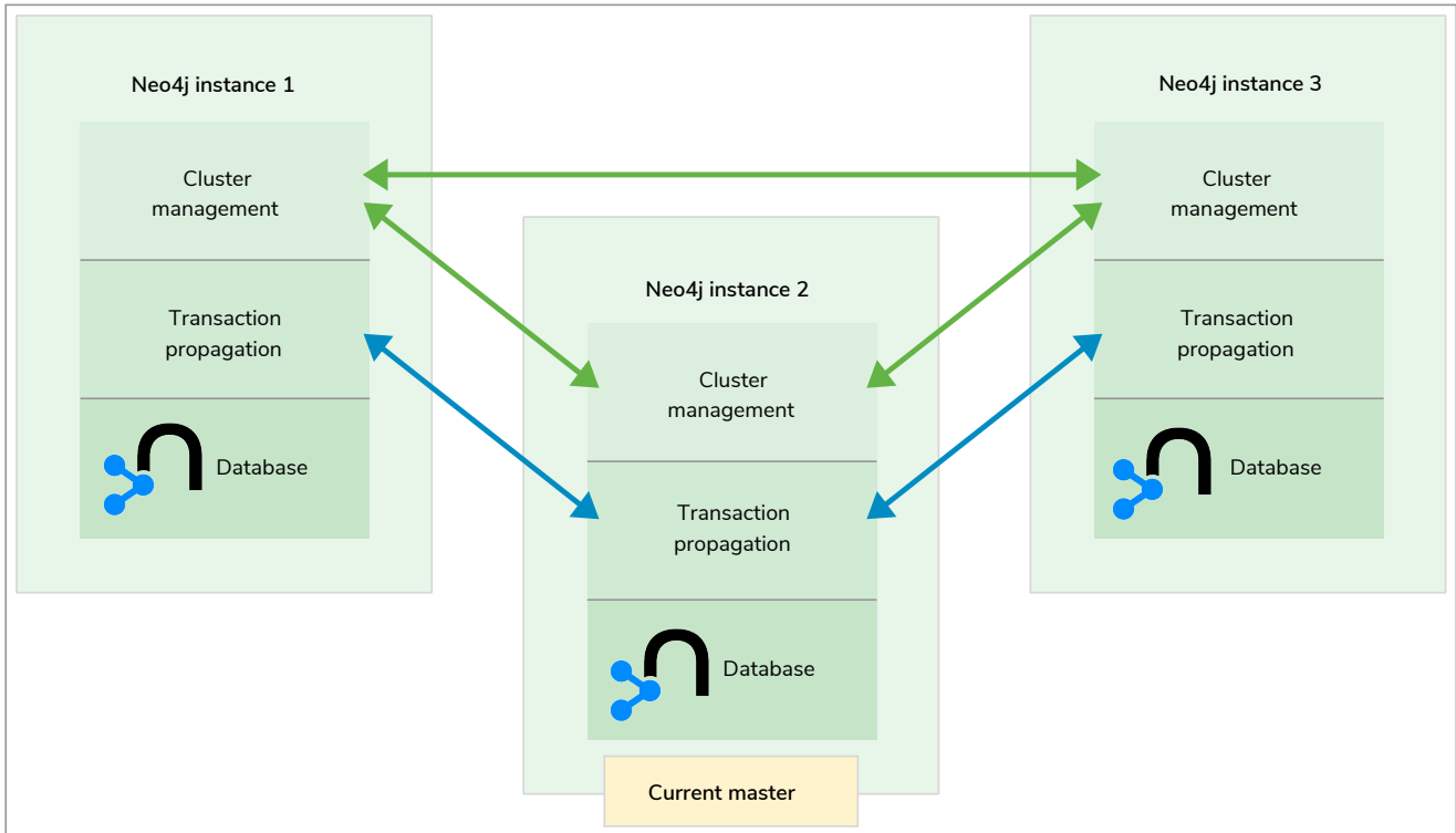
Figure 24. A Neo4j HA cluster
